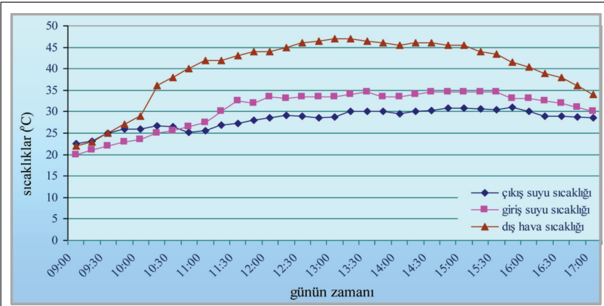
Şekil 8. Dış Hava Sıcaklığına Bağlı Olarak Kolektör Giriş-Çıkış Suyu Sıcaklıkları İlişkisi
