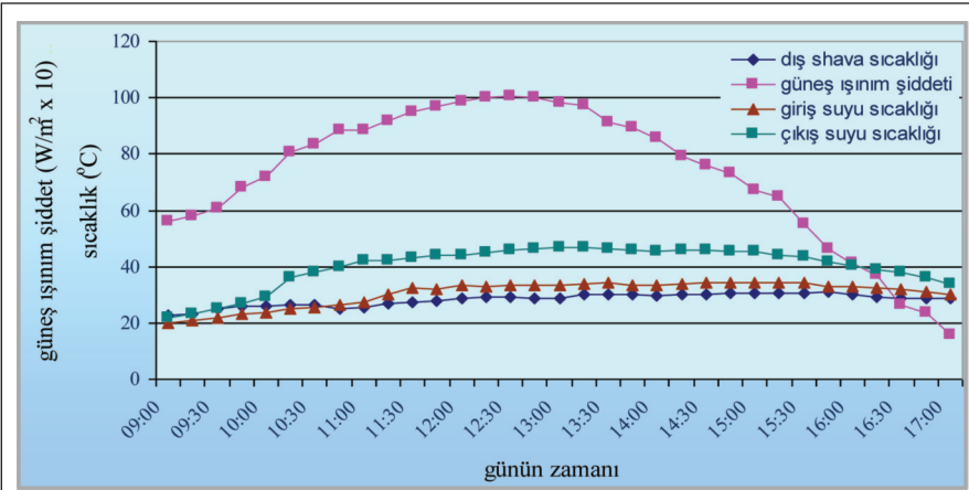
Şekil 9. Dış Hava Sıcaklığı ve Güneş Işınım Şiddetine ve Kolektör Giriş-Çıkış Suyu Sıcaklıkları İlişkisi
