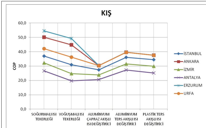
Şekil 13. Kış Koşullarında Çeşitli Isı Değiştiricilerin COP Değerleri
