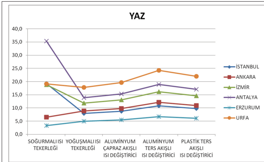
Şekil 12. Yaz Koşullarında Çeşitli Isı Değiştiricilerin COP Değerleri
