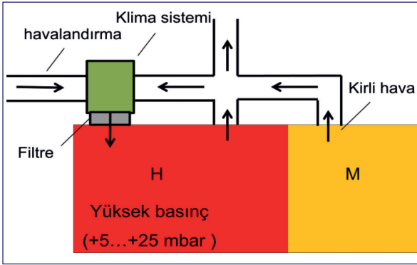
Şekil 5. Kontrollü Şekilde Yönlendirilmiş Hava Akımı (Tek Yönlü) [4]
