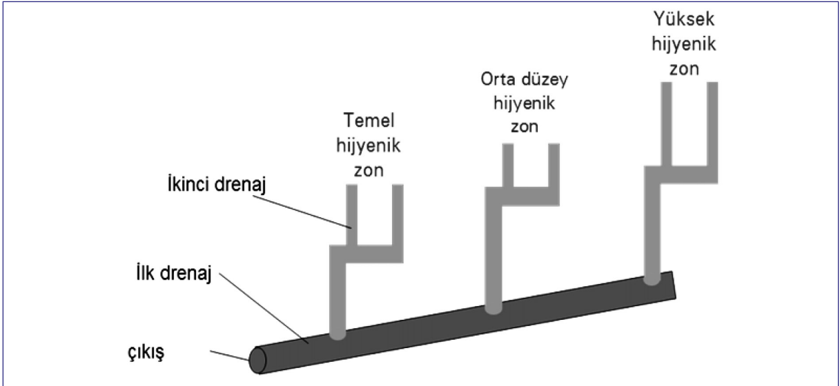
Şekil 1. Atık ve Yan Ürün Hareketliliği [4]
