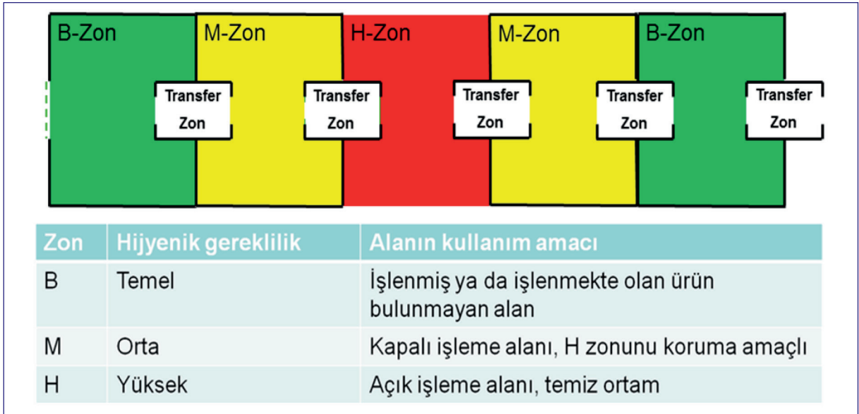
Şekil 3. Hijyen Alanlarının Jenerik Yerleşimi [4]
